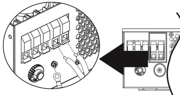
PV 5000MH
